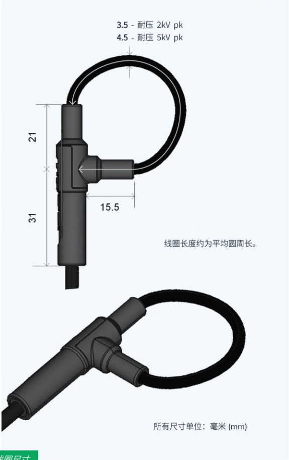
线圈尺寸
